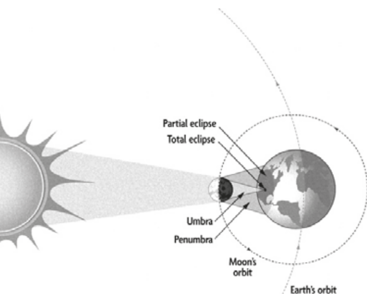
Geometría de un eclipse solar
