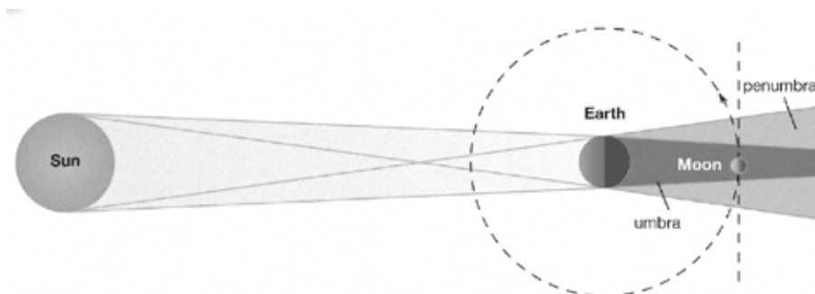
Geometría de un eclipse lunar
